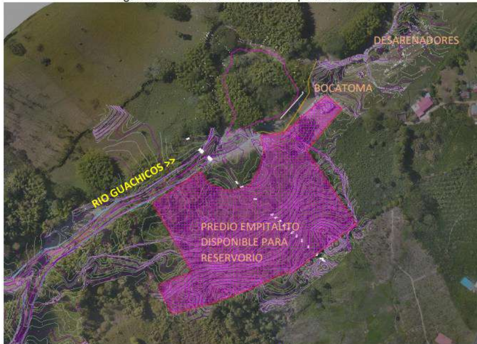
Figura 14. Predio de EMPITALITO ESP para reservorio
